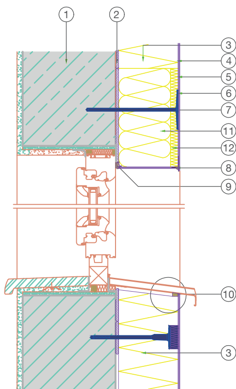
Detajl
